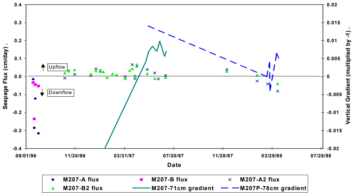
a. ENR Seepage Flux --M207
